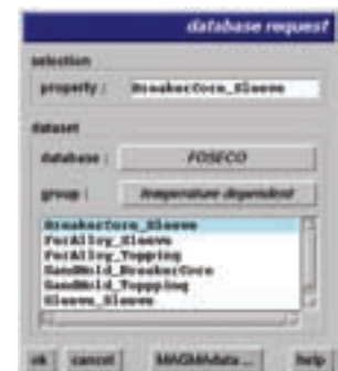
Database dei coefficienti di trasferimento del calore specifici dei prodotti FOSECO
