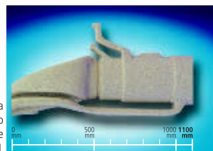
Anima complessa per getti in alluminio con agglomerante POLITEC AL
